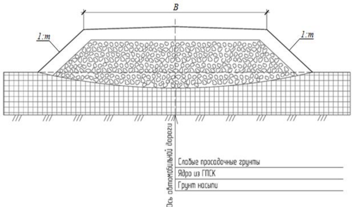
Рисунок 5 – Поперечный профиль насыпи с теплоизоляционным материалом –гранулированной пеностеклокерамикой совместно с нетканым геотекстилем при проектировании насыпей по 1-му принципу
